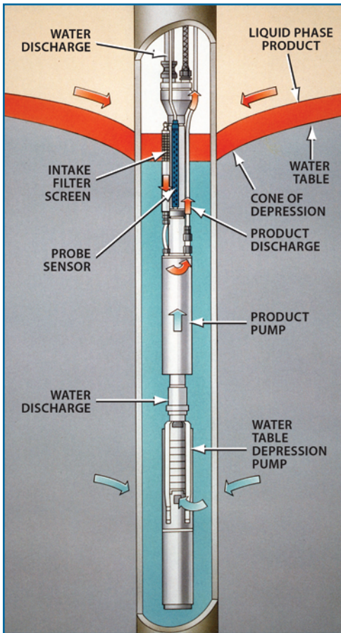
小直径探针清扫机 和地下水抽水泵联用示意图
