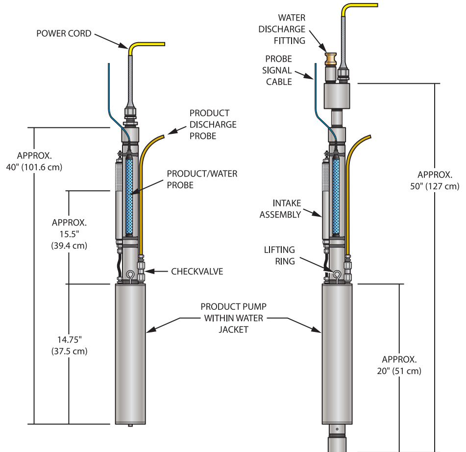
单独工作组装图
