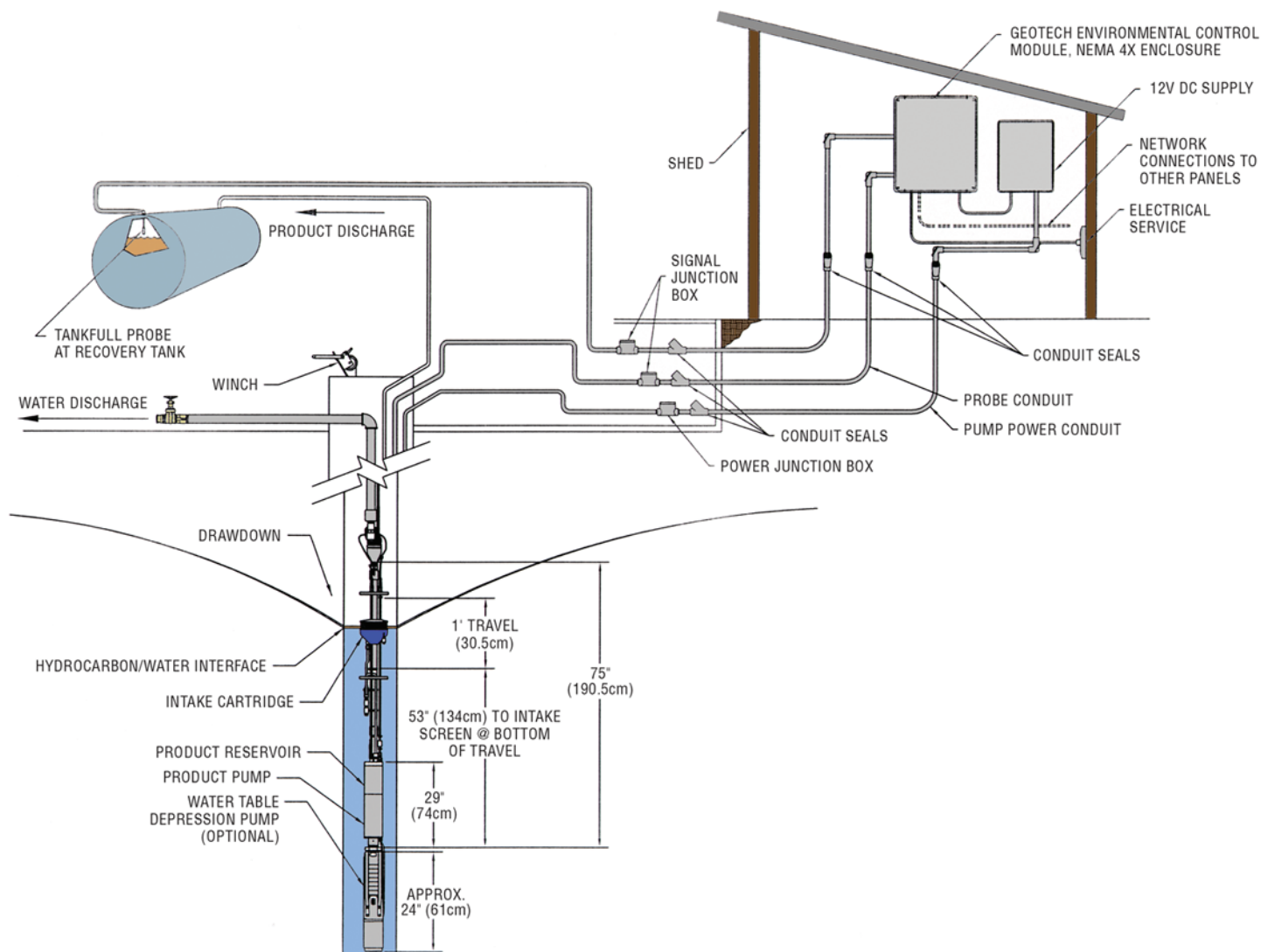
典型配置：小直径过滤式清理器™ 和地下水减压泵系统
