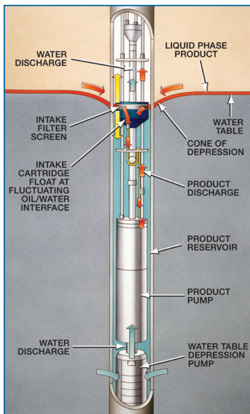
井下作业示意图
