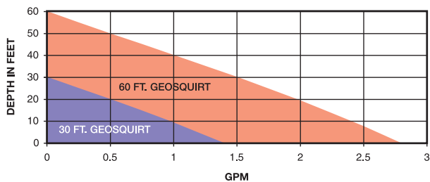
geosquirt™ 工作曲线
