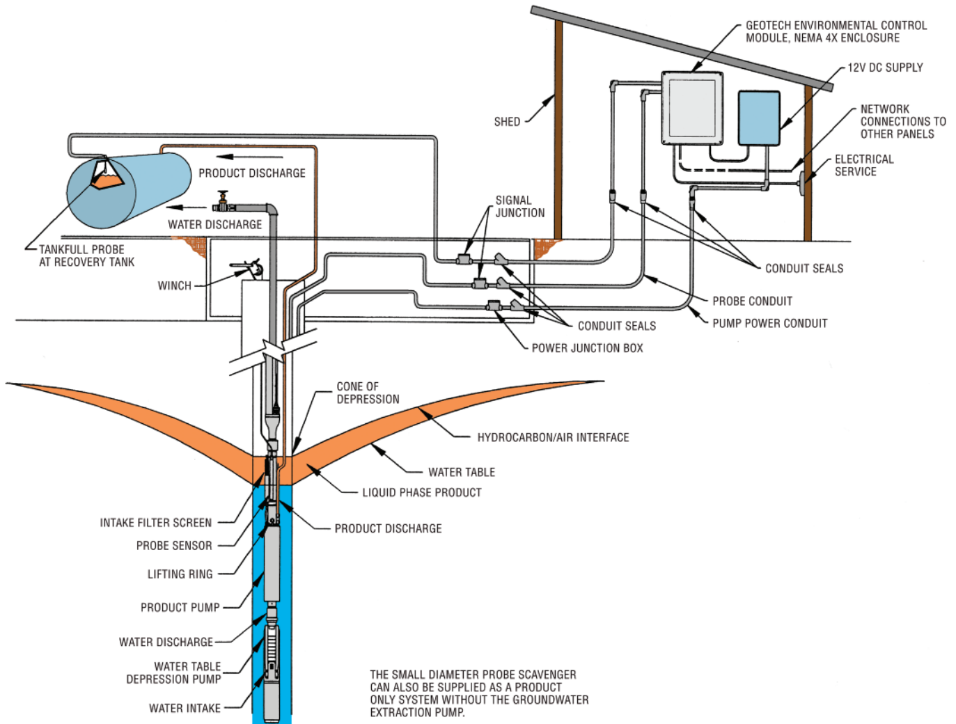
Geotech Small Diameter Probe Scavenger™ 碳氢化合物回收系统
