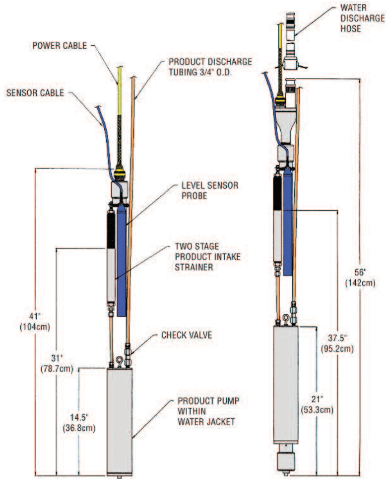
单独工作组装图
